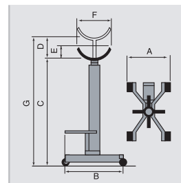
ГАБАРИТЫ / DIMENSIONS / ABMESSUNGEN DIMENSIONS / DIMENSIONI (мм)
